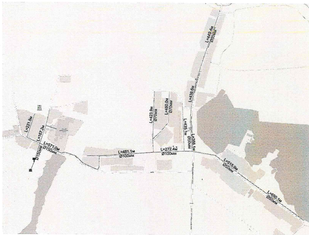
Рис.6 - Схема водоснабжения д. Пронь, д. Дудкино, д. Новоселки
