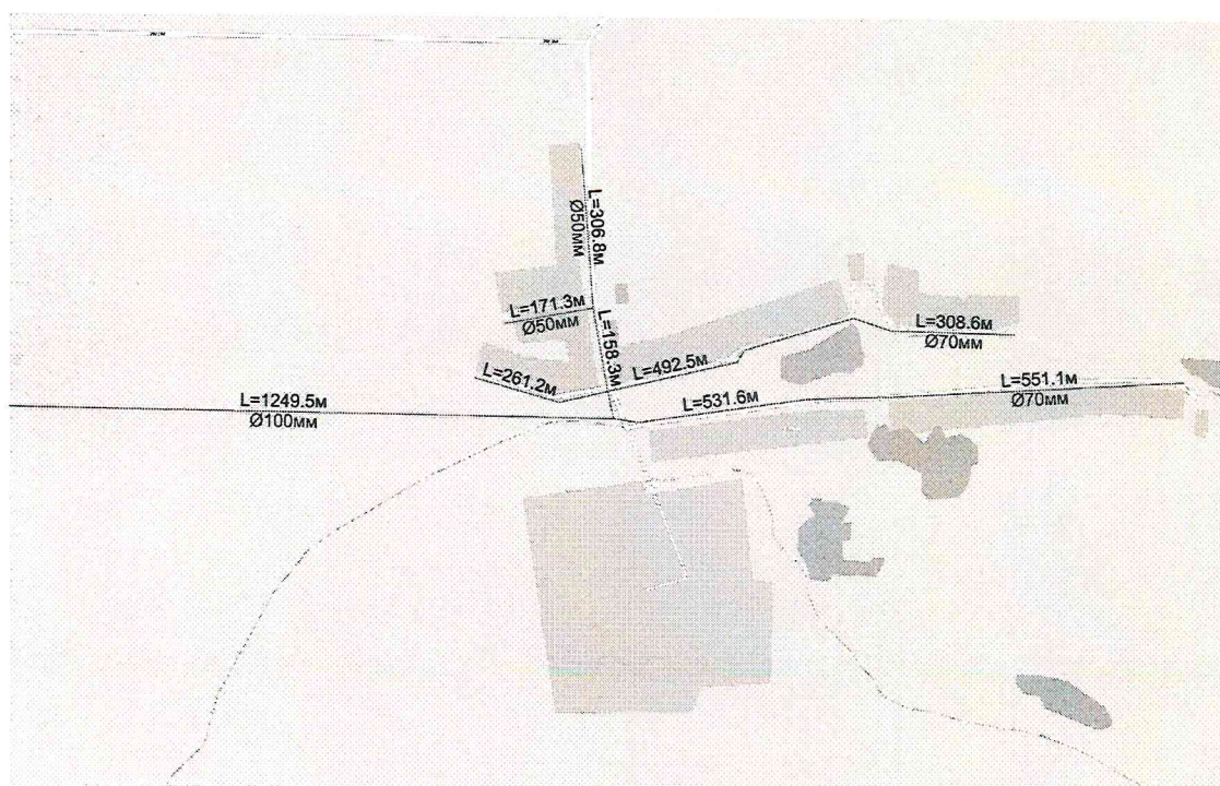
Рис.7 - Схема водоснабжения д. Zubovka
