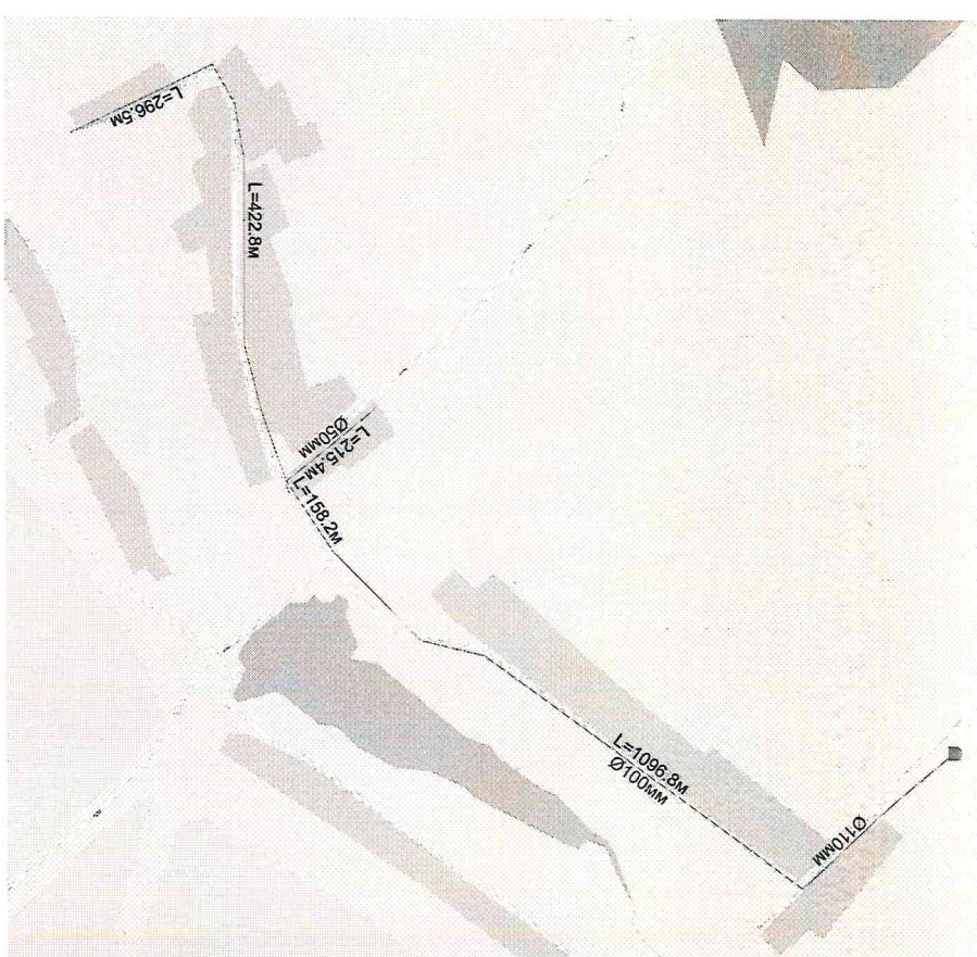
Рис.5 - Схема водоснабжения с. Транкино
