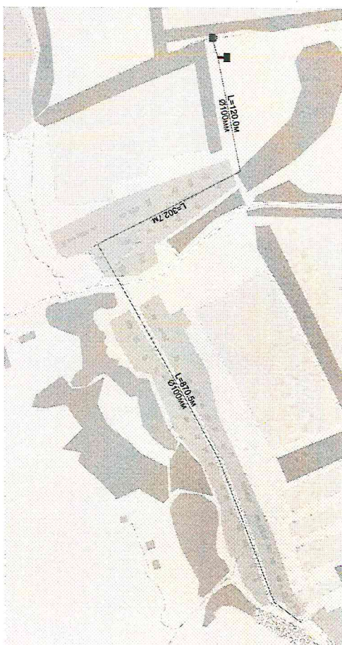
Рис.3 - Схема водоснабжения д. Алексеевка
